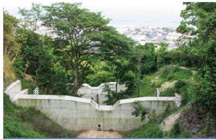
治山ダム（完成時）上流側
